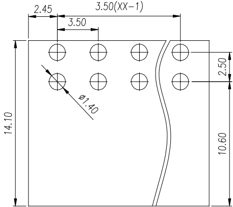
P.C.B. LAYOUT
